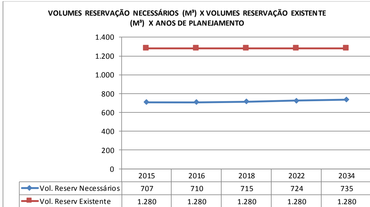
Gráfico 3.3 – Volumes de Reservação Necessários (m 3 ) x Volume de Reservação Existente (m 3 ) x Anos de Planejamento
